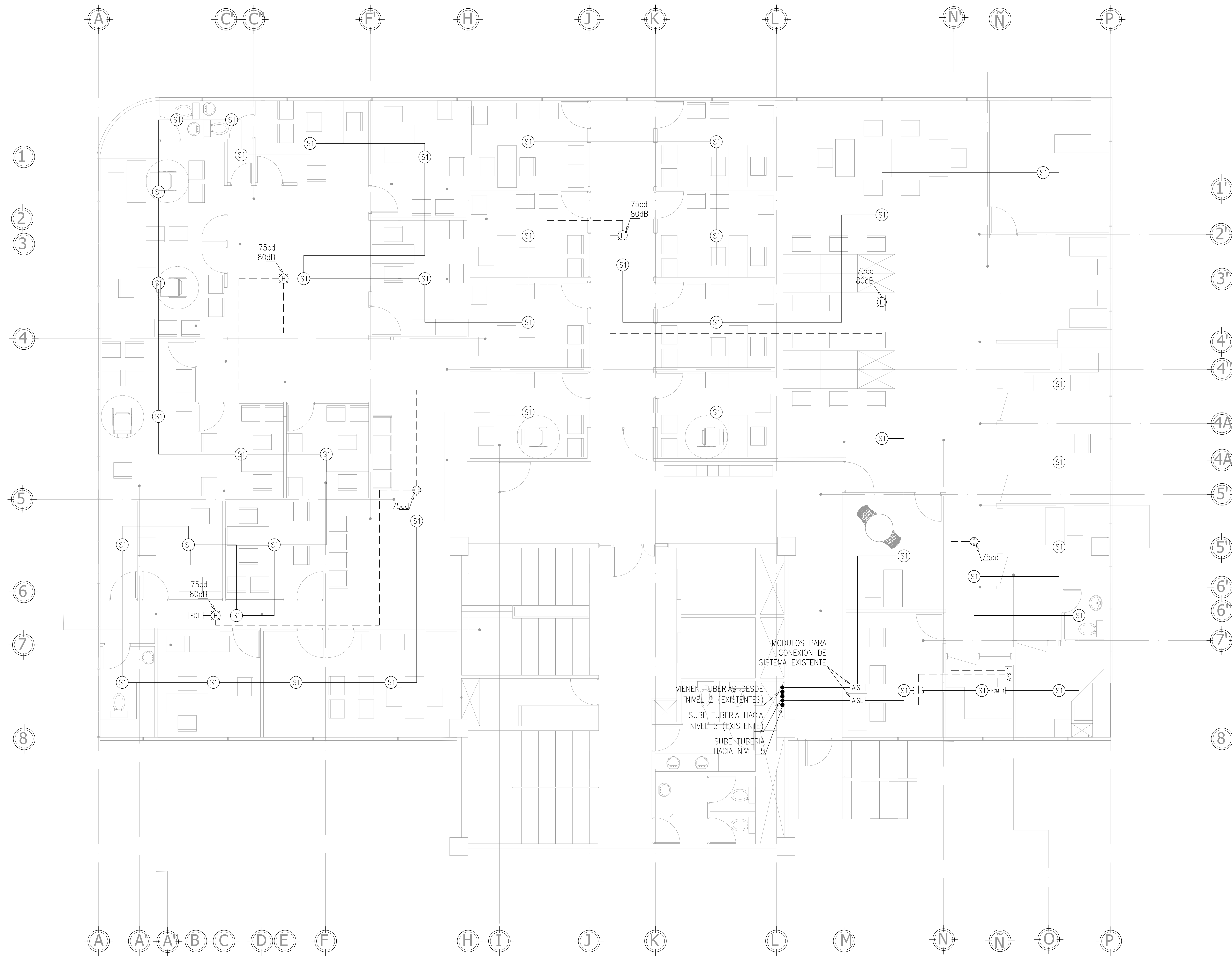
PLANTA DE DETECCION DE INCENDIOS NIVEL 3 ESCALA 1:50
