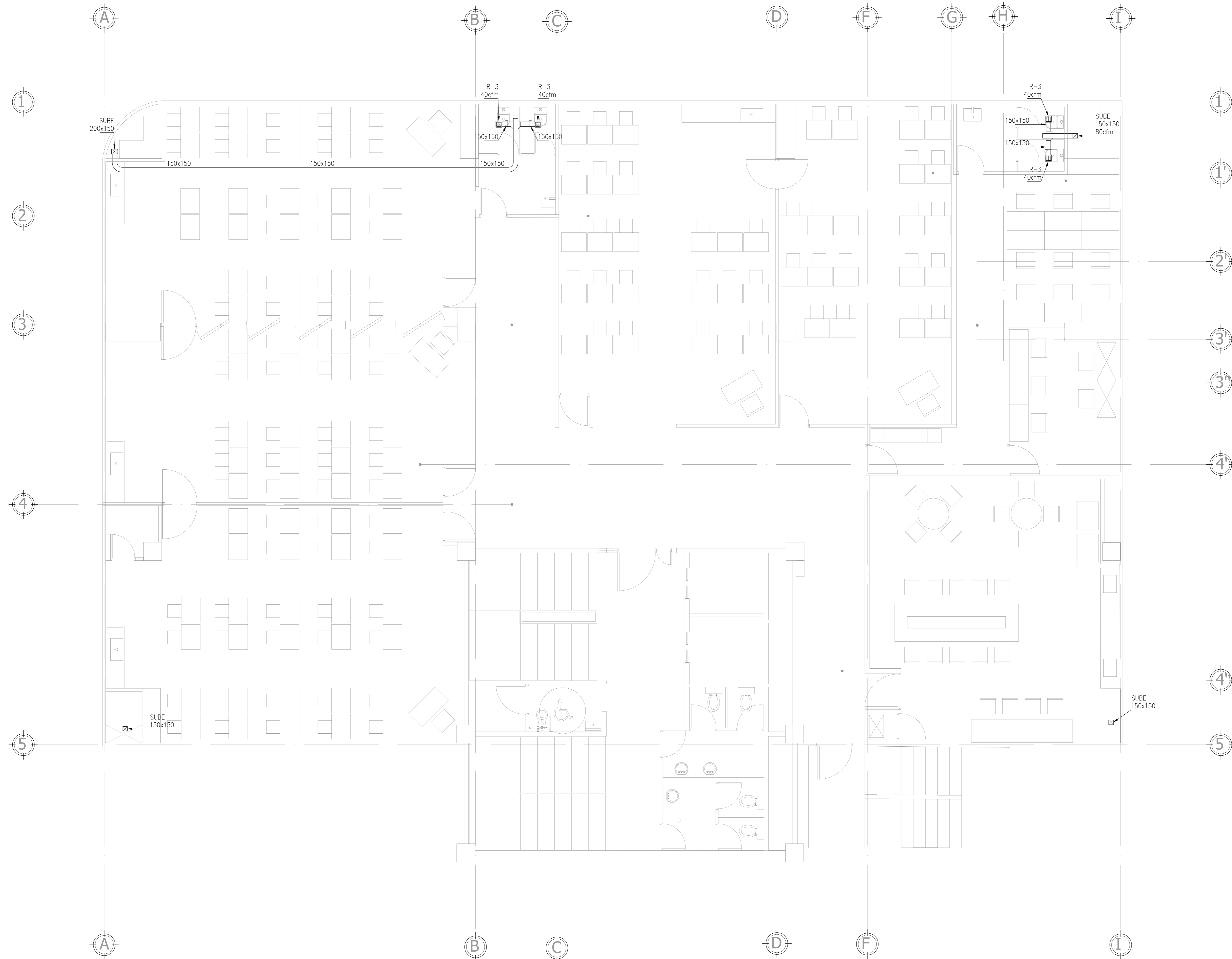
PLANTA DE EXTRACCION NIVEL 5 ESCALA 1:50
